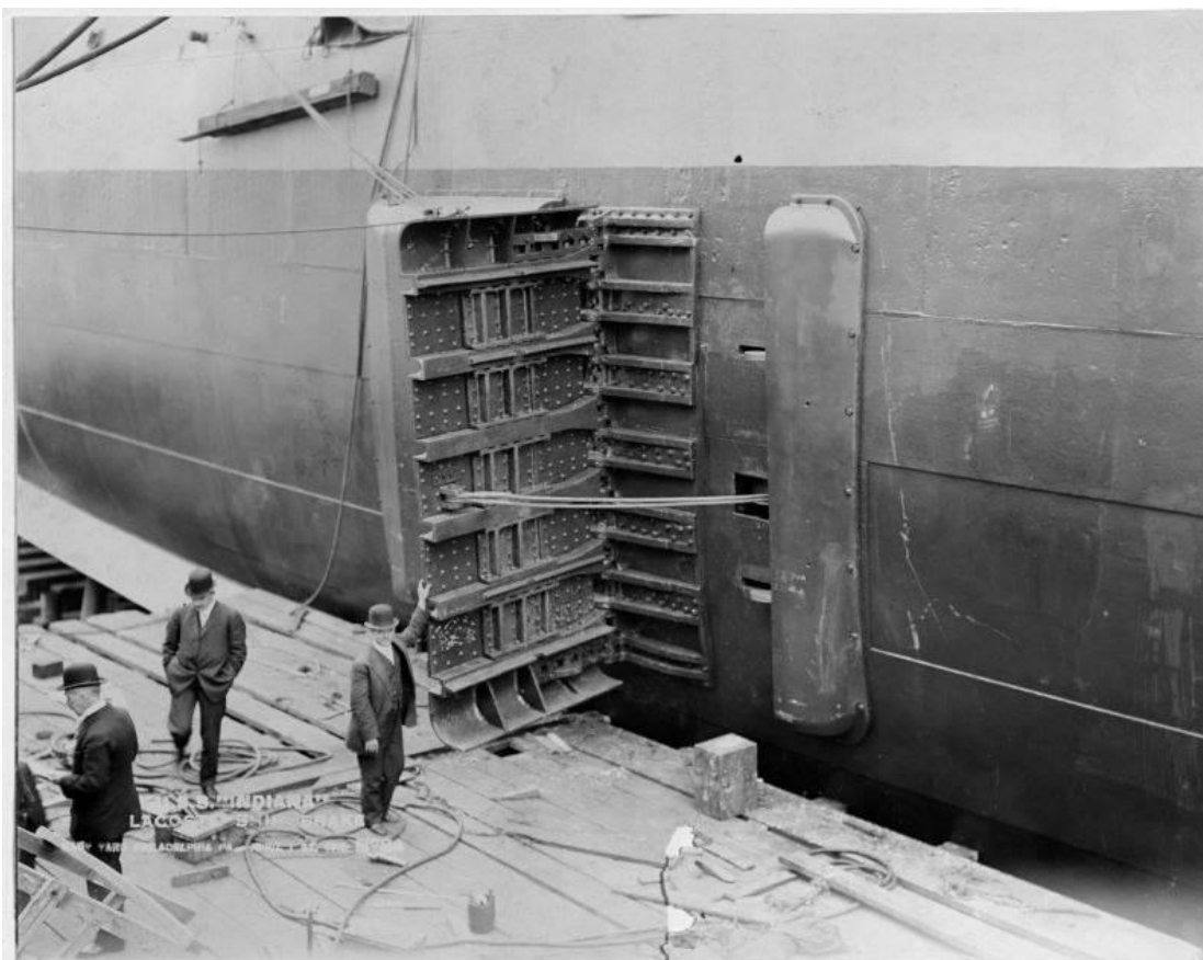
Freno hidrodinámico del Iowa
